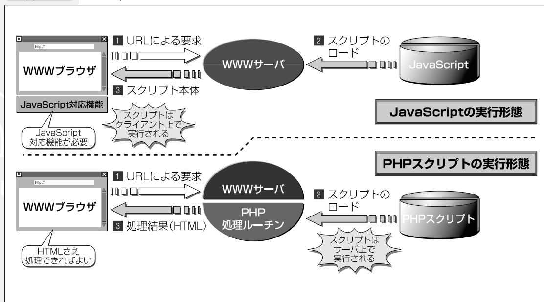
図 1-5 JavaScript と PHP
